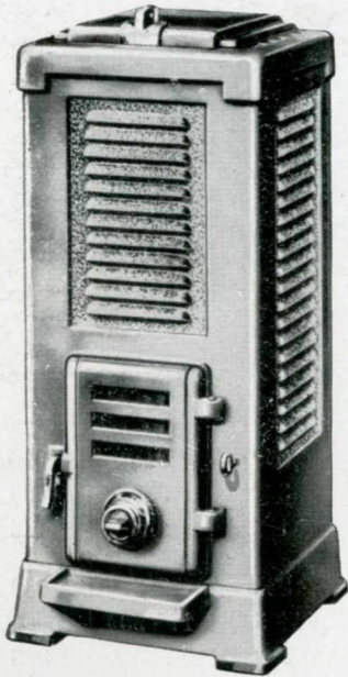
Calorifères " DÉVILLE AÉROTOL " à tirage direct
