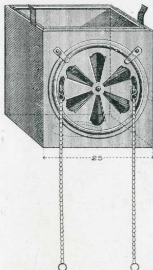
Chapiteau tôle galvanisée
