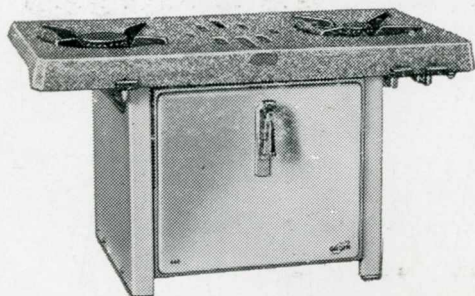
Fourneau "Four Godin" N° 440 à deux brûleurs "Clasen" sur le dessus, brûleur breveté "Trio" dans le four.
